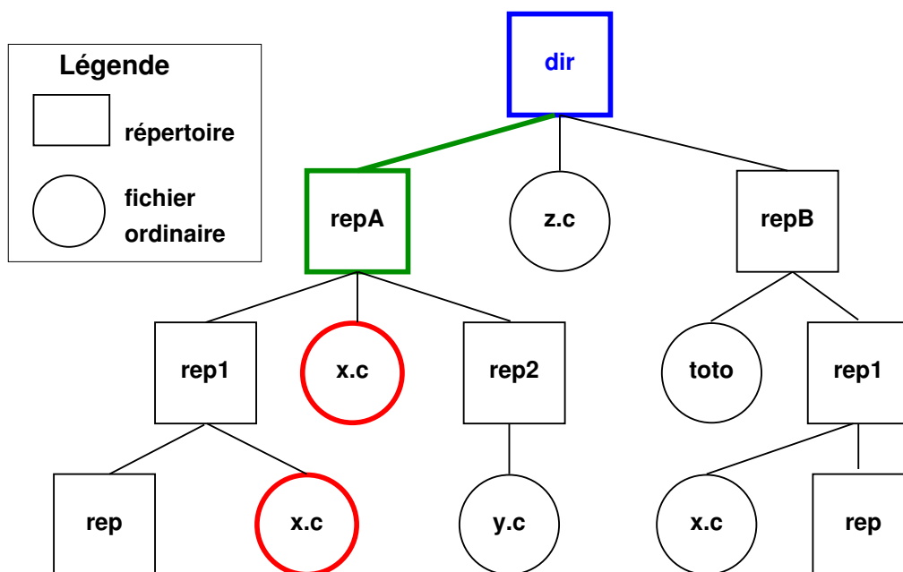
FIGURE 3.8 – Si dir est le répertoire de travail, la commande qui permet de rechercher les fichiers nommés x.c dans la branche partant du sous-répertoire repA est find repA -name x.c -print
