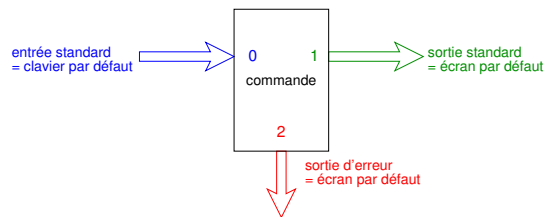
FIGURE 10.1 – Flux standard de données associés à une commande
